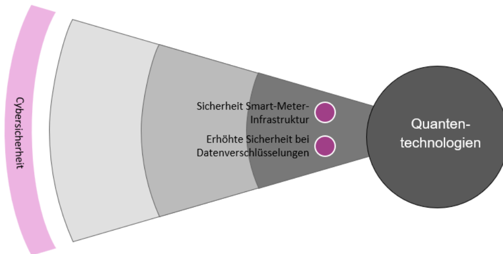
Abbildung 9: Anwendungsfälle „Cybersicherheit“
