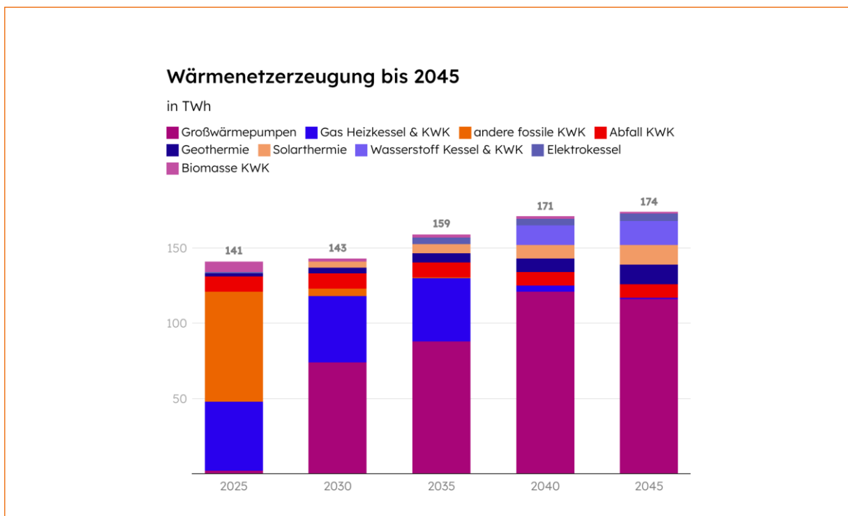
Abbildung 1: Wärmeerzeugung in deutschen Wärmenetzen bis 2045 (Quelle: LFS, Szenario T45–Strom) i
