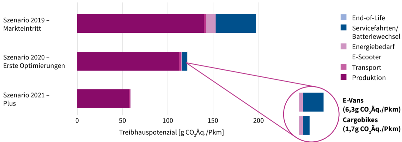
Abbildung 6: Treibhauspotenzial des E-Scooter-Sharings bezogen auf einen Personenkilometer für die betrachteten Nutzungs- und Betriebsszenarien, Quelle: dena
