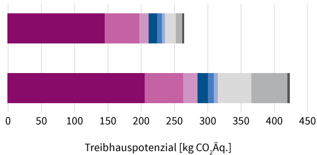
Abbildung 4: Treibhausgasemissionen in der Produktionsphase der Referenz-E-Scooter, Quelle: dena
