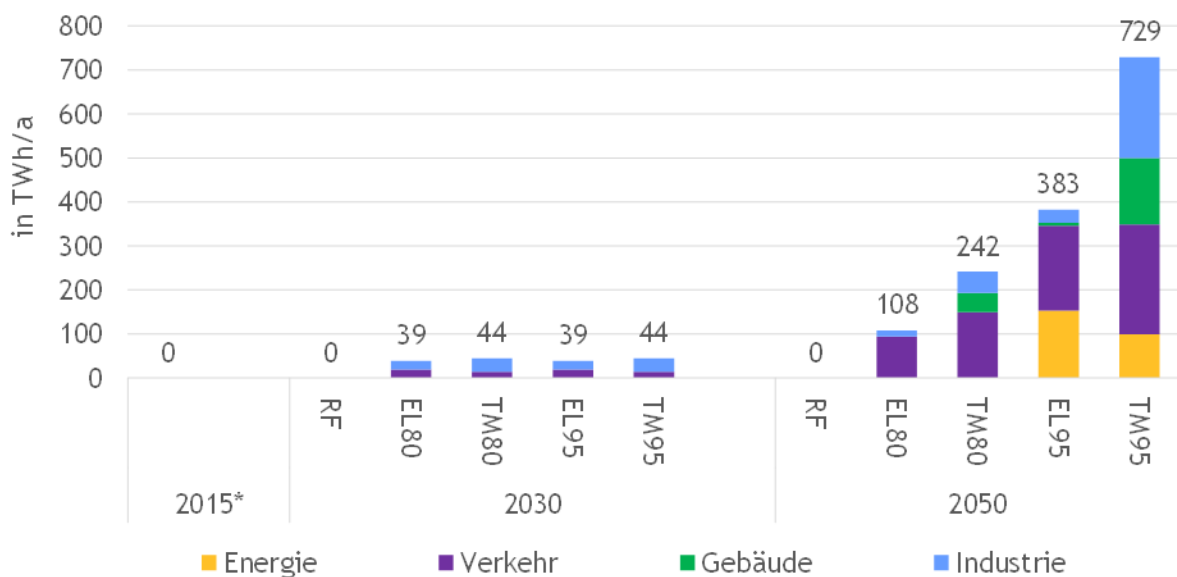
Abb. 13: Endenergieeinsatz von PtX in Deutschland nach Sektor [in TWh/a] 17
